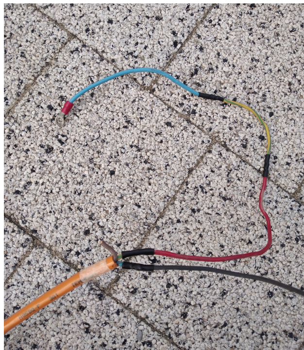
Fot. 11 Po 40 latach główny kabel zasilający składał się z 7 odcinków
