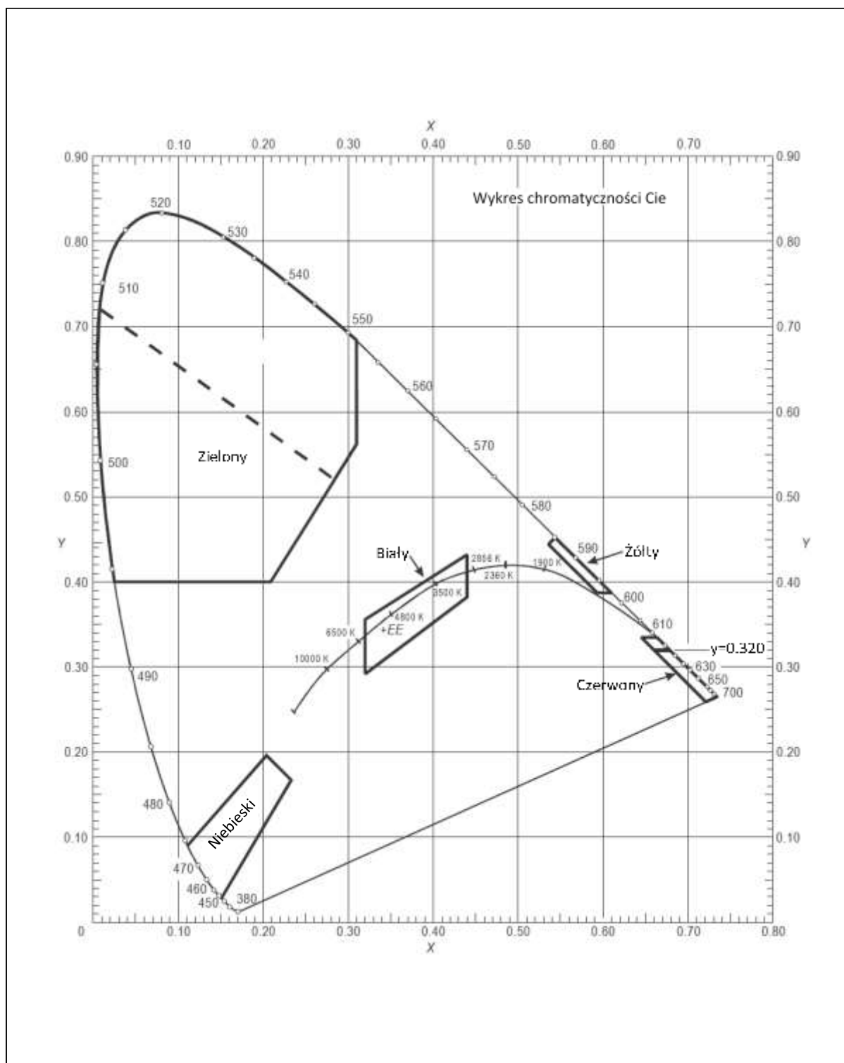
Rysunek A1-1b. Kolory naziemnych światel lotniczych (światła o charakterze stałym)
